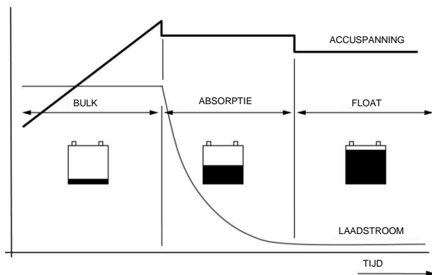
Afbeelding 6: 3-trapslaadproces
