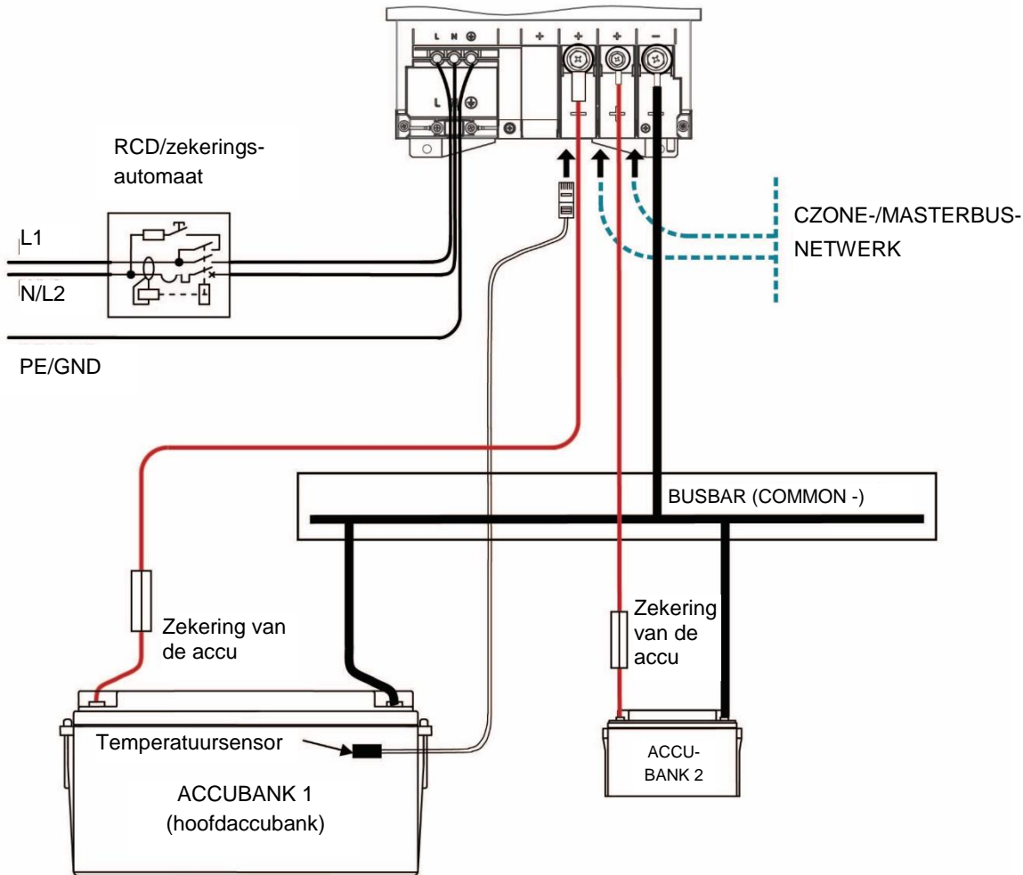
Afbeelding 3: Installatietekening van de ChargeMaster Plus
