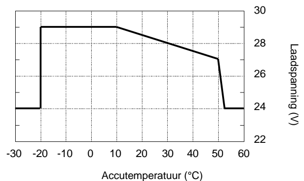
Afbeelding 7: Temperatuurgecompenseerd laden
