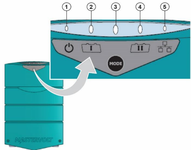
Afbeelding 5: ChargeMaster Plus Statusleds
