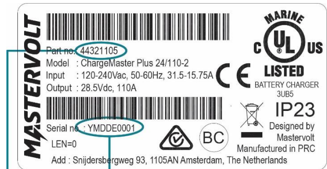
Afbeelding 1: Identificatiesticker
